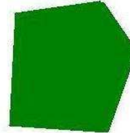
Pentágono no regular
